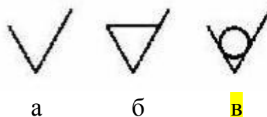
Рис. 1. Обозначение шероховатости
