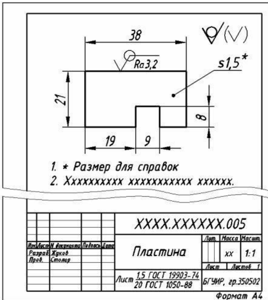
Рис. 3. Чертеж детали с одинаковой шероховатостью поверхностей, образующих контур
