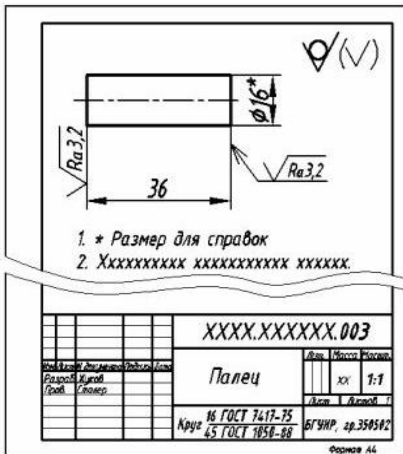
Рис. 2. Чертеж детали с поверхностью, которая по данному чертежу не обрабатывается
