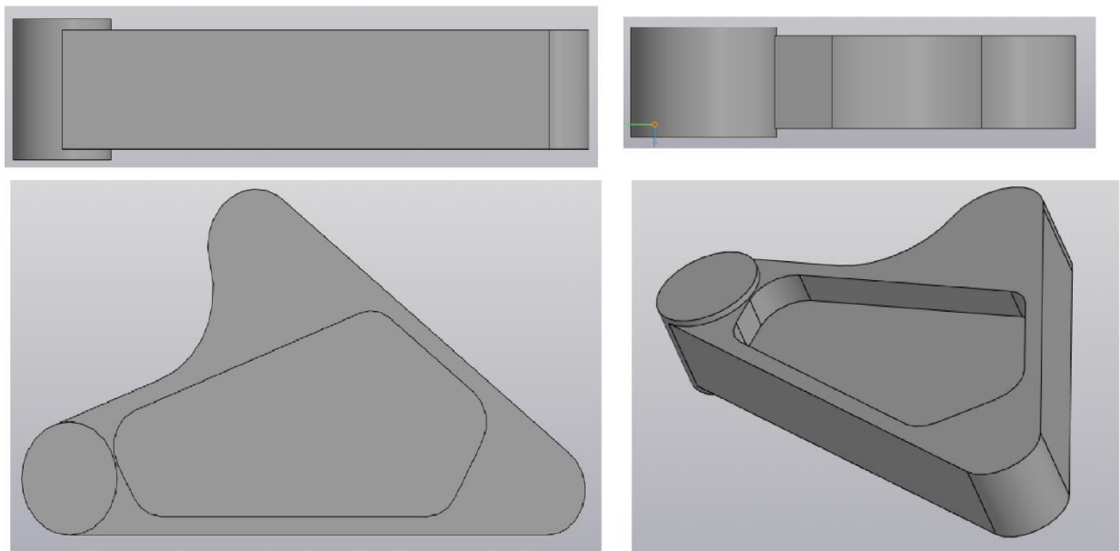
Рисунок 1.3 – Комп'ютерна 3D-модель заготовки деталі «Качалка»
