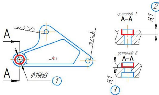
025 4214 «Вертикально-свердлильна»
