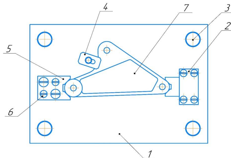
Рисунок 2.2 – Схема кондуктора: 1 – плита кондуктора ; 2 – призма рухома; 3 – направляючі колони; 4 – притиск; 5 – призма; 6 – гвинти; 7 - деталь
