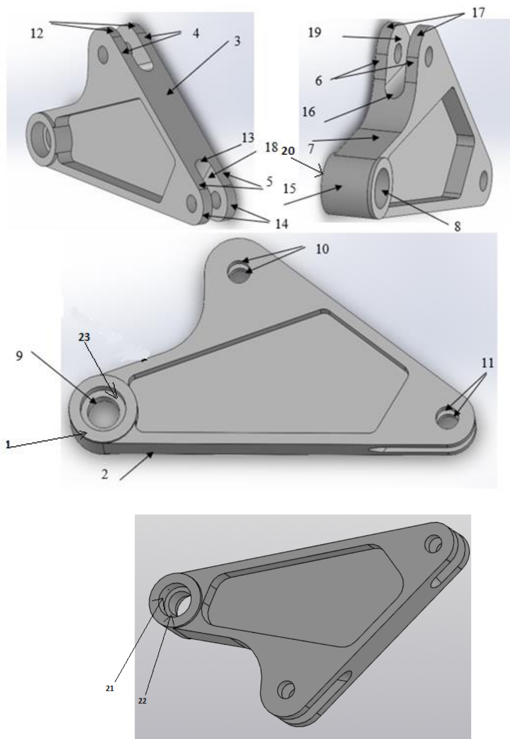
Рисунок 1.2 – Позначення оброблюваних поверхонь деталі «Качалка»
